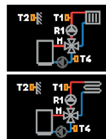
Schéma s 4-cestným ventilem
